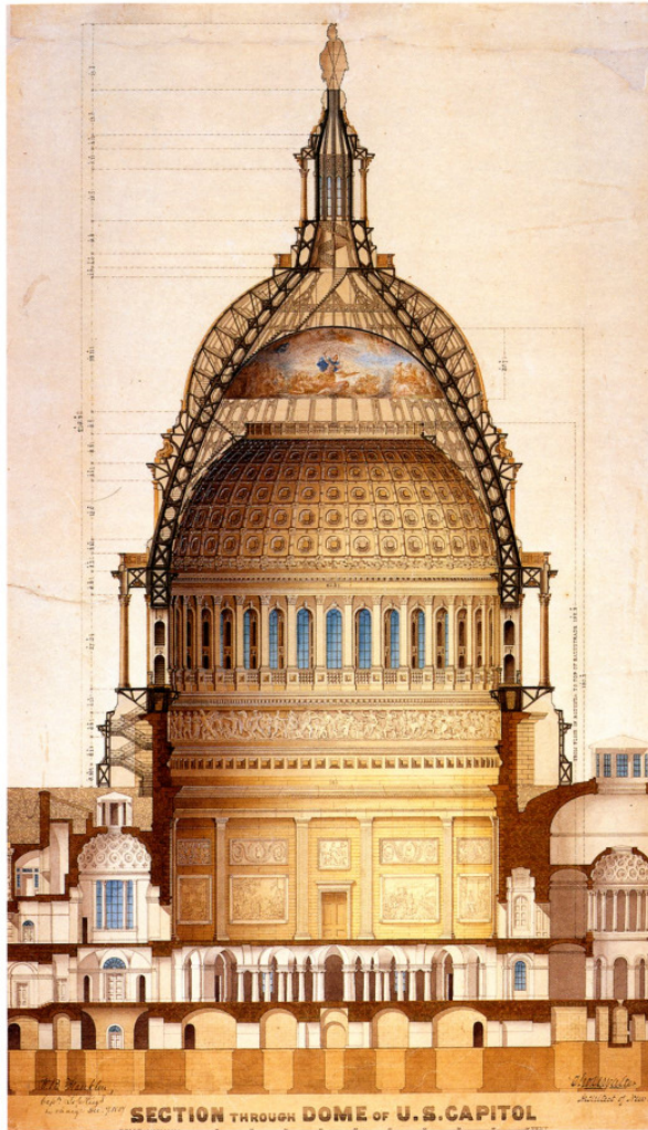
Abb. 6: Schnitt durch die Kuppel des Capitol
